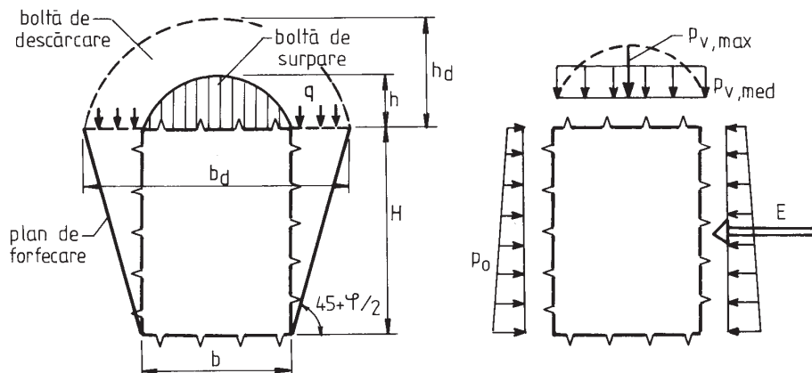
Figura nr.12. Notații pentru relațiile de calcul
