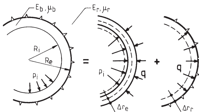
Figura nr.17. Definierea reacțiunii elastice a rocii
