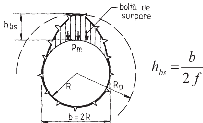
Figura nr.8. Formarea boltii de surpare
